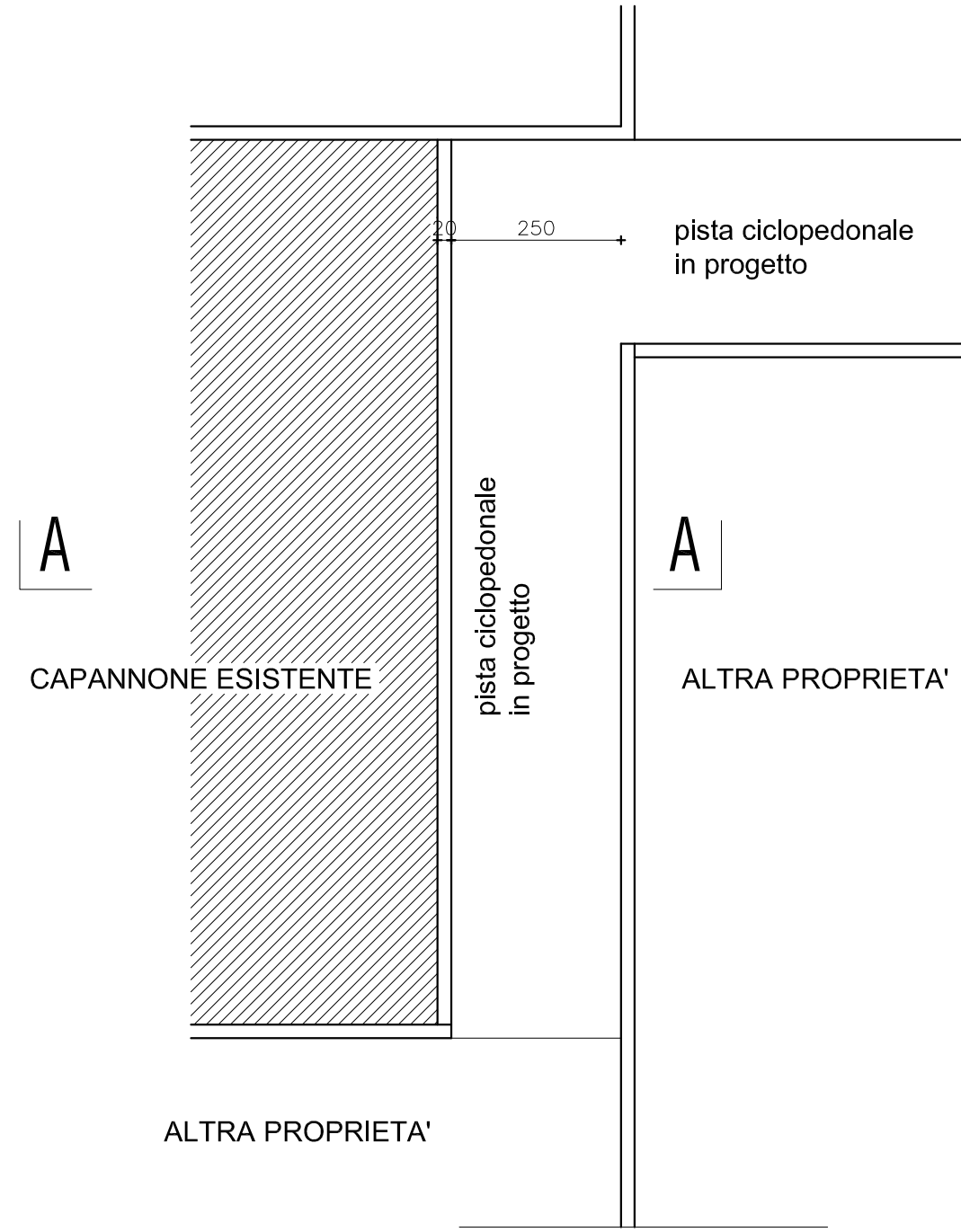
PIANTA - Progetto
