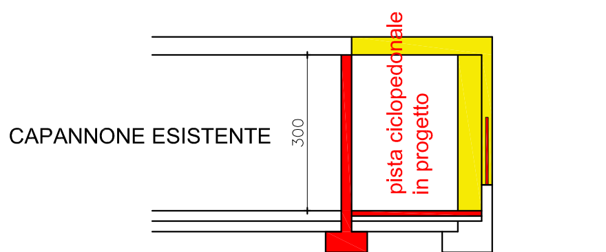
SEZIONE - Individuazione interventi
