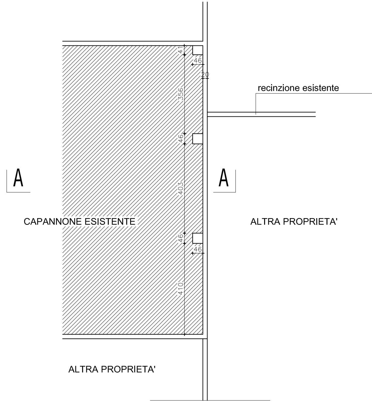
PIANTA - Stato di fatto
