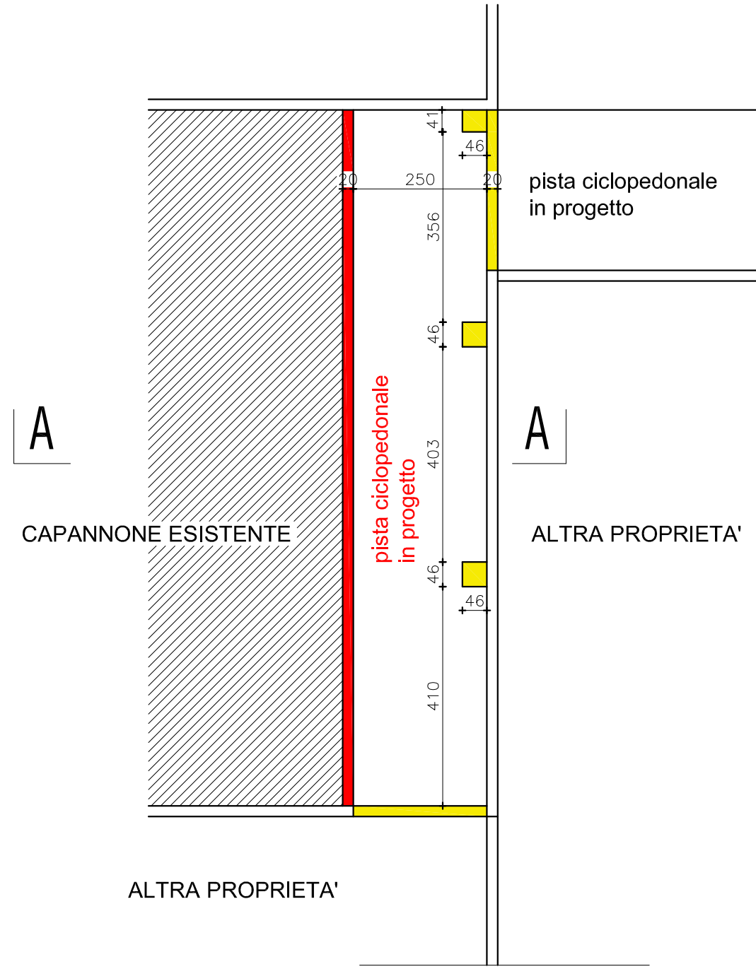
PIANTA - Individuazione interventi
