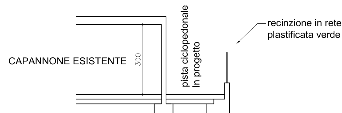
SEZIONE - Progetto
